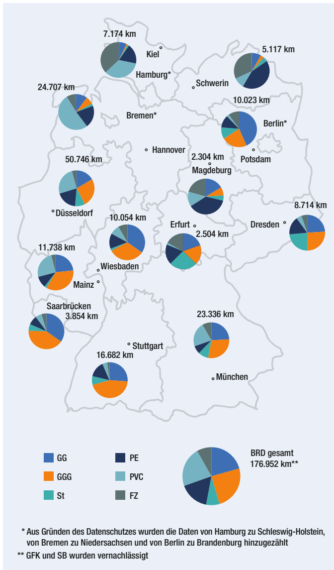
Abbildung 3 Prozentuale Verteilung der eingesetzten Materialien von Versorgungsleitungen nach Bundesländern mit Angabe der ausgewerteten Länge 2
